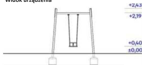
Widok urządzenia
