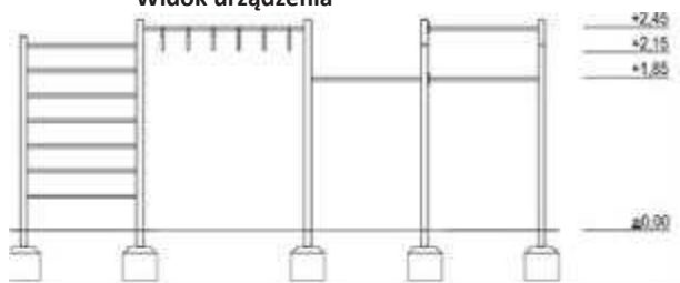
Widok urządzenia
